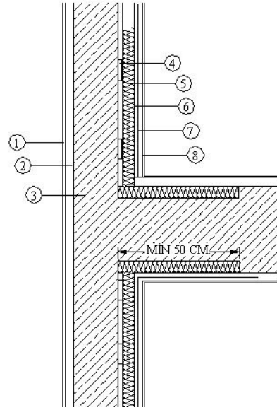
B- İÇTEN YALITIM
