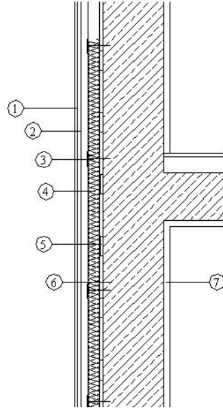
A- DIŞTAN YALITIM
